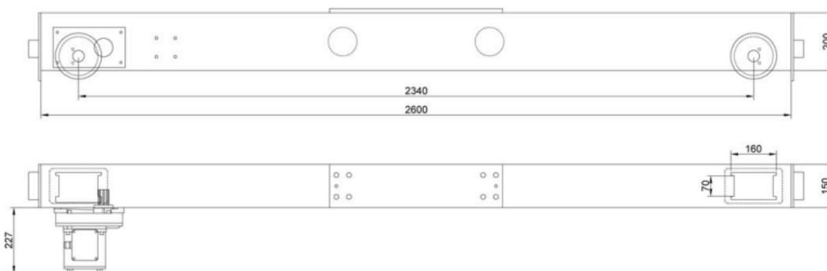
1048263 Балка концевая опорная TOR г/п 3,0 т 2,6 м (Т)
