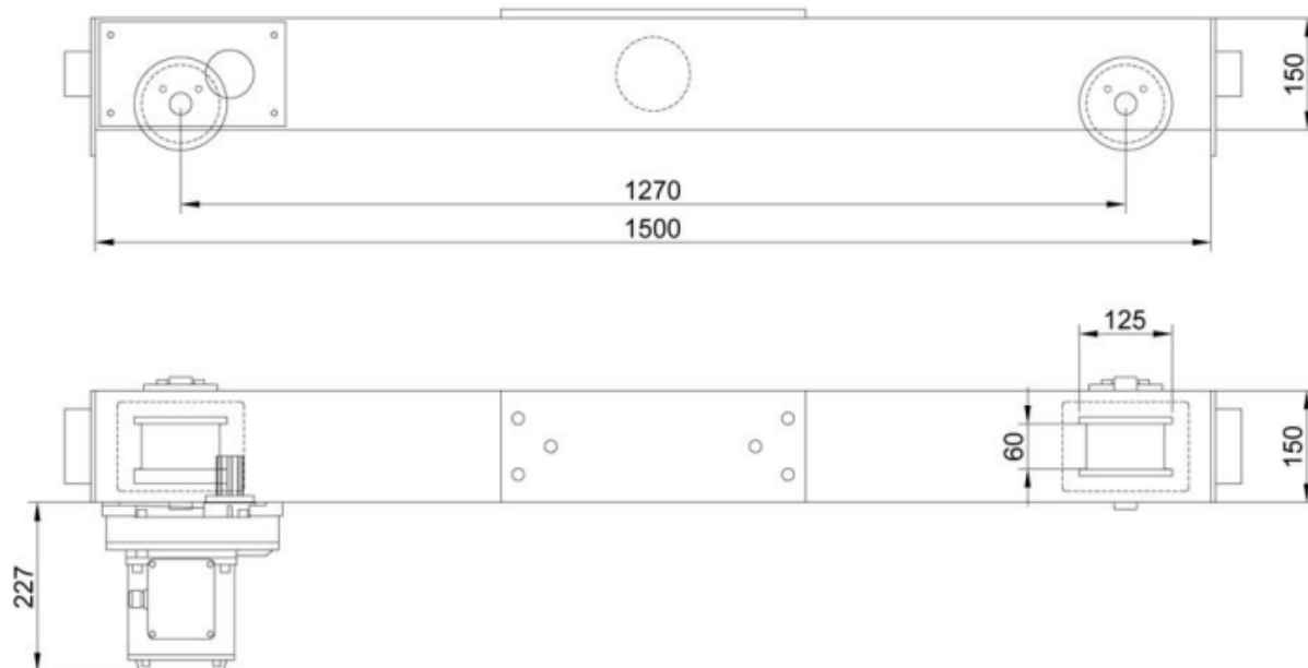
1048259 Балка концевая опорная TOR г/п 2,0 т 1,5 м (Т)
