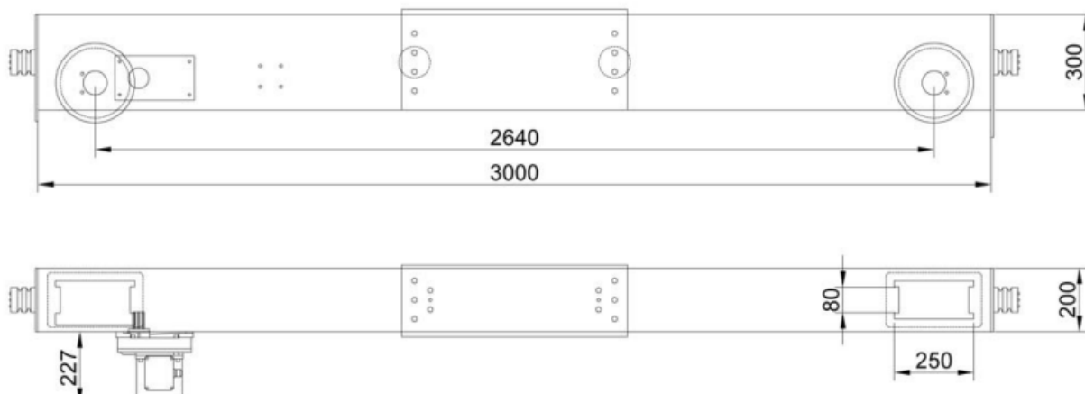
1048491 Балка концевая опорная TOR г/п 10,0 т 3,0 м (Т)
