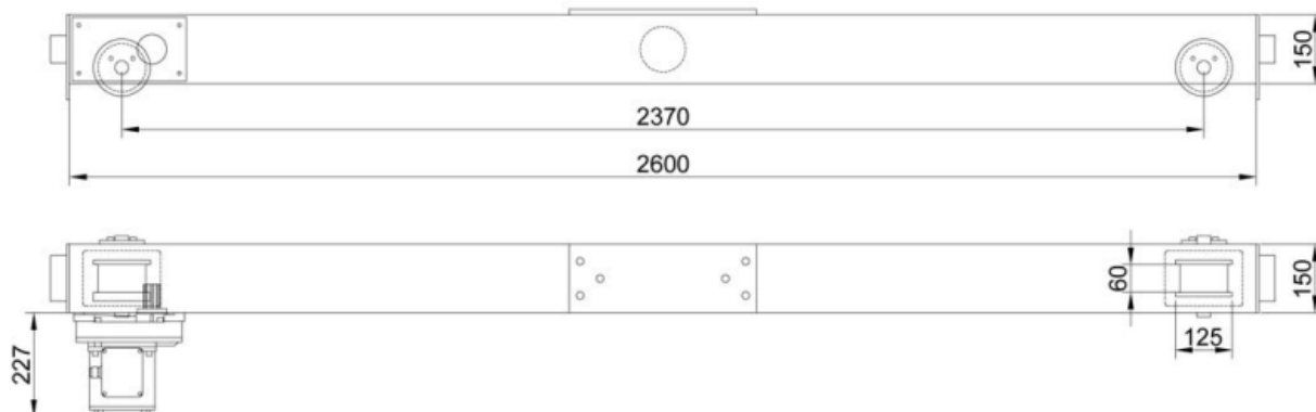
1048968 Балка концевая опорная TOR г/п 2,0 т 2,6 м (Т)
