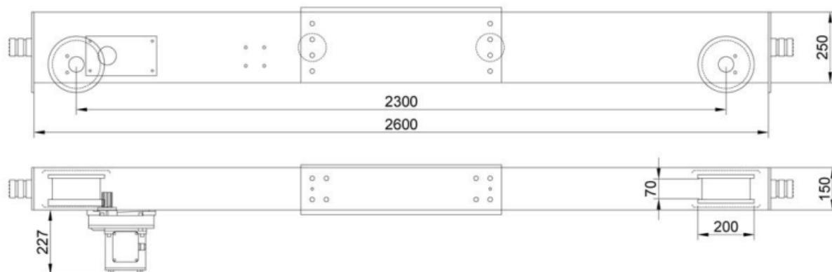
1048492 Балка концевая опорная TOR г/п 5,0 т 2,6 м (Т)
