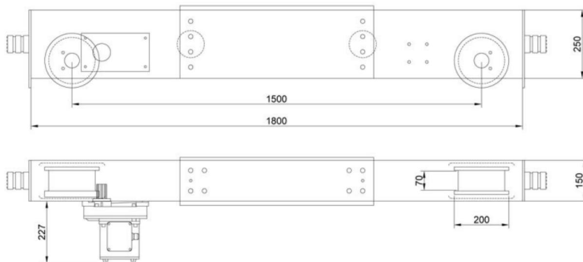
1048969 Балка концевая опорная TOR г/п 5,0 т 1,8 м (Т)
