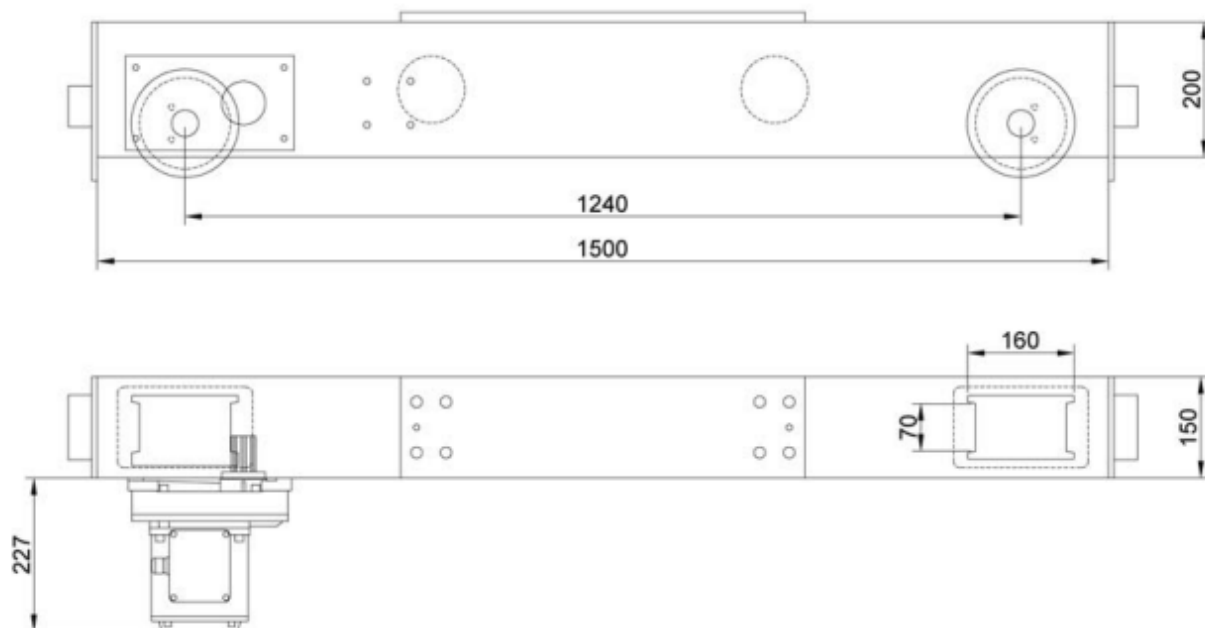
1048260 Балка концевая опорная TOR г/п 3,0 т 1,5 м (Т)
